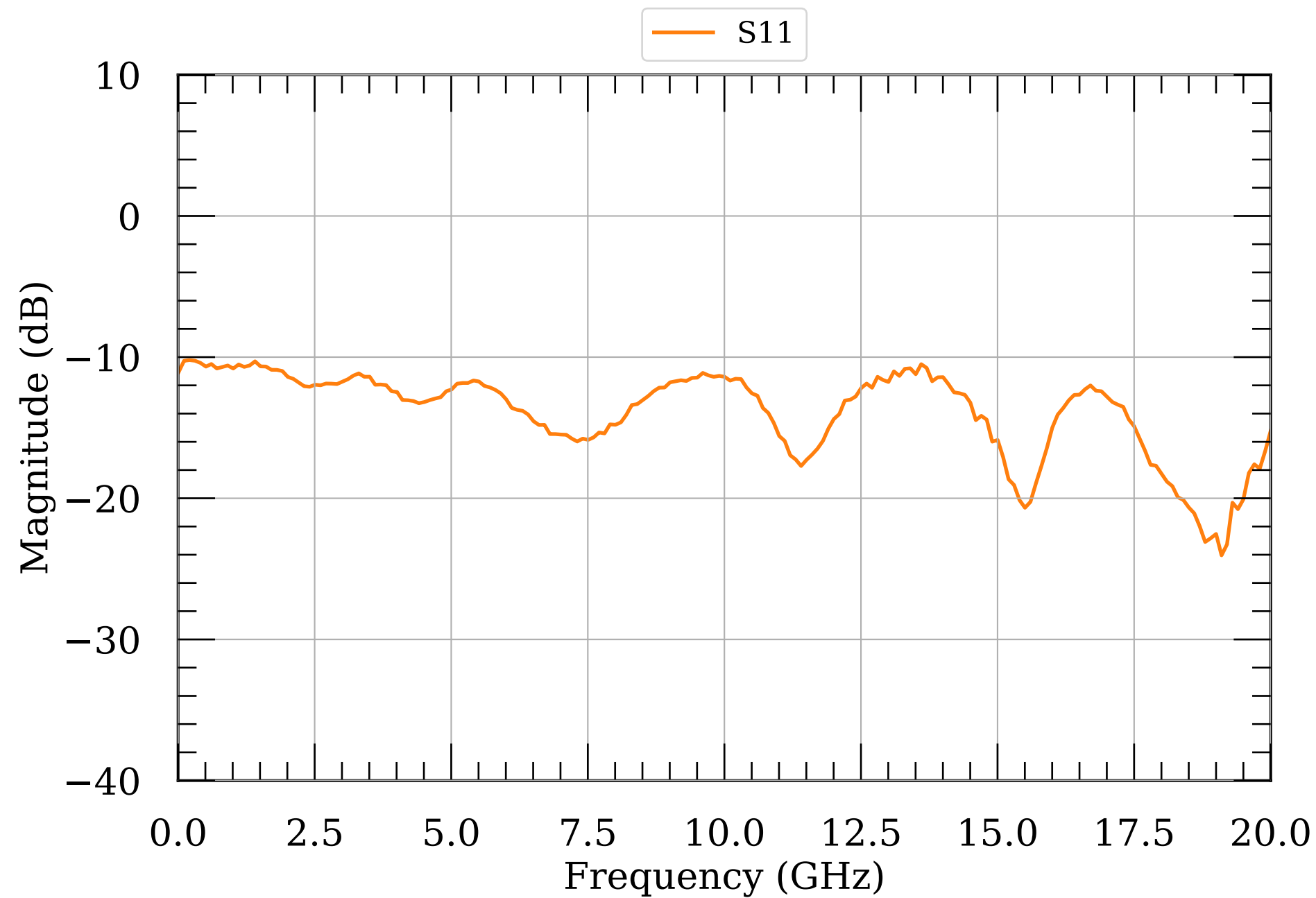
LNA S-params module044
